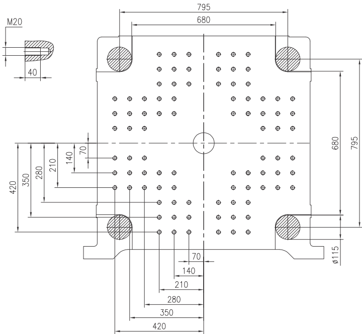
Fixed platen 定模板
