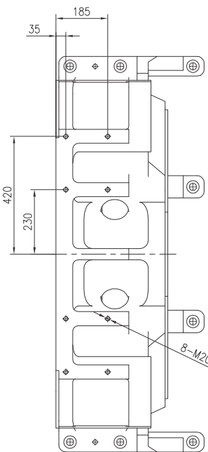
Fixed platen 定模板
