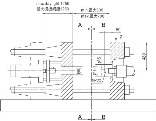
Movable platen 动模板
